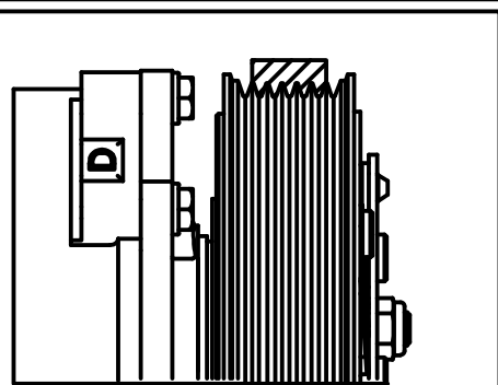
Схема расположения ремня на шкиве компрессора SD5H14
